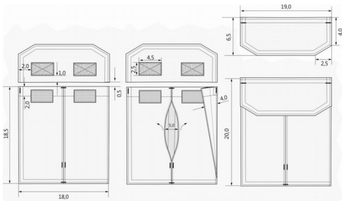
1.5 - Detalhes do bolso cargo
