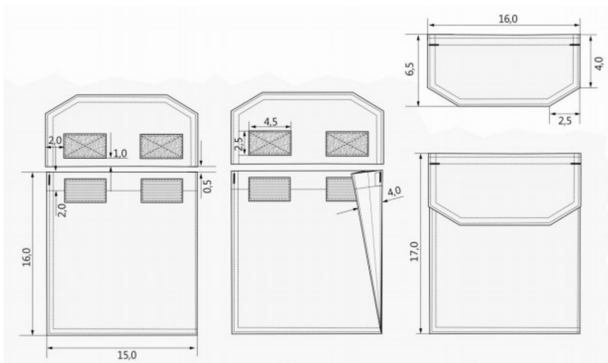
1.7 – Detalhes da braguilha e do pertingal
